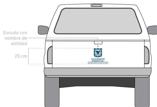
Vista posterior
