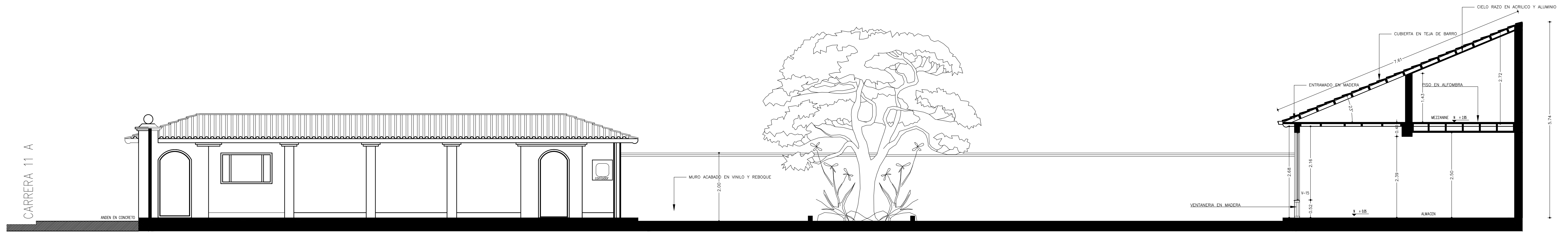
CORTE FACHADA PORTERIA ESCALA 1:50
