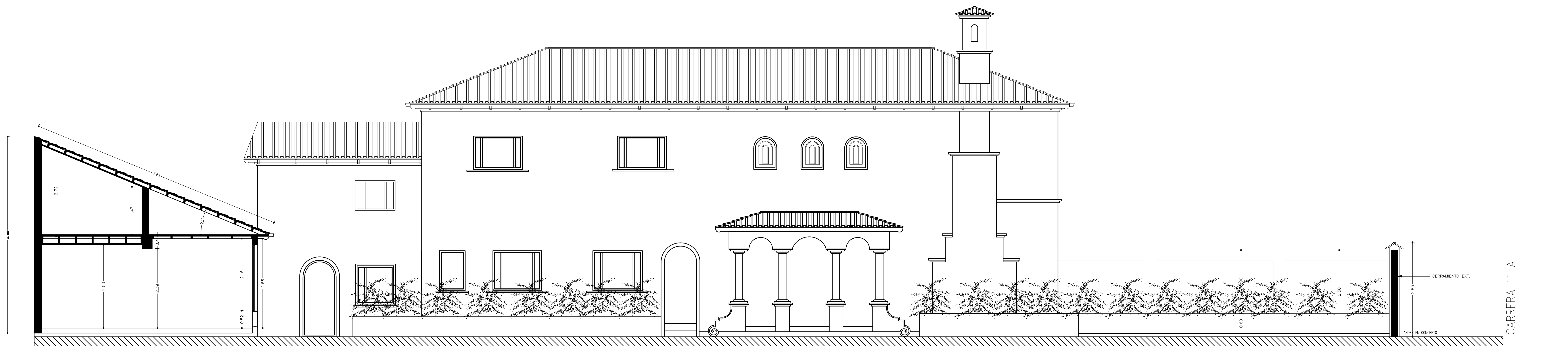
CORTE FACHADA ACCESO PPAL ESCALA 1:50
