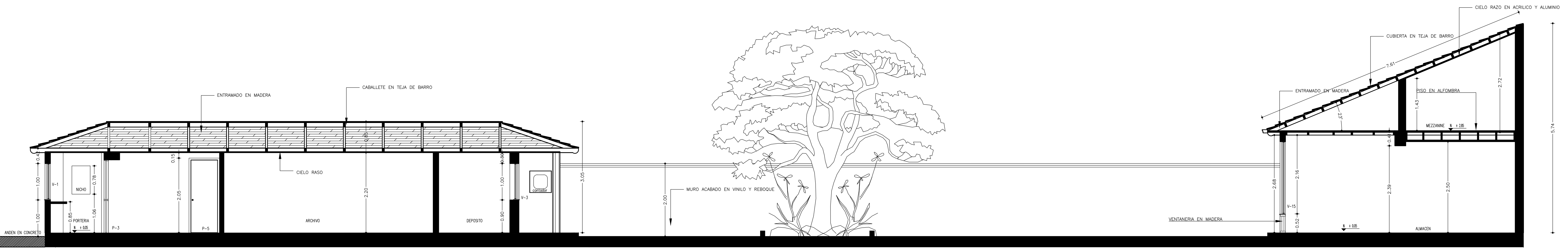
CORTE A-A ESCALA 1:50
