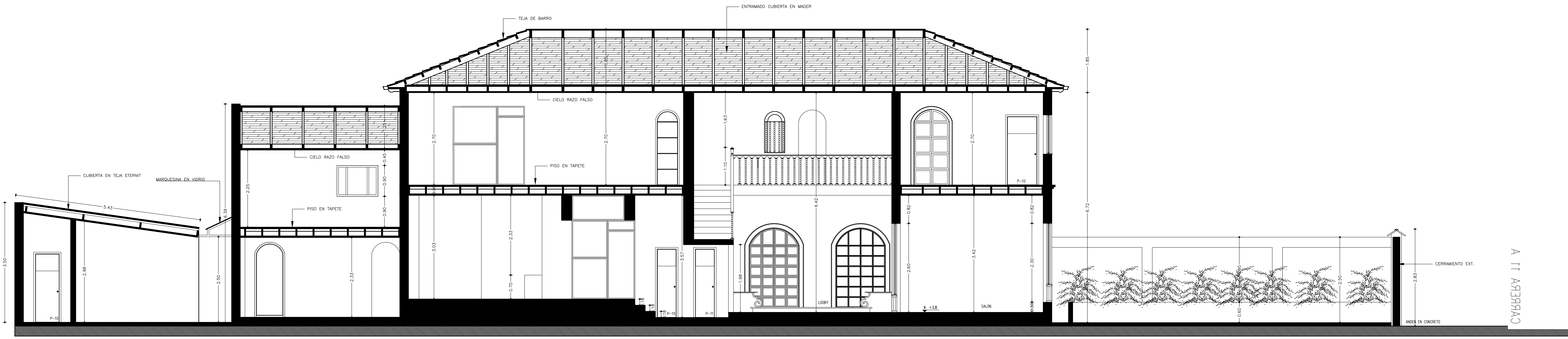
CORTE B-B ESCALA 1:50
